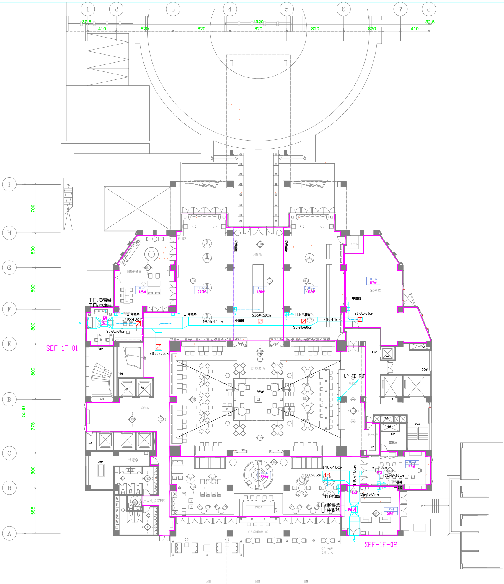
壹層平面圖
