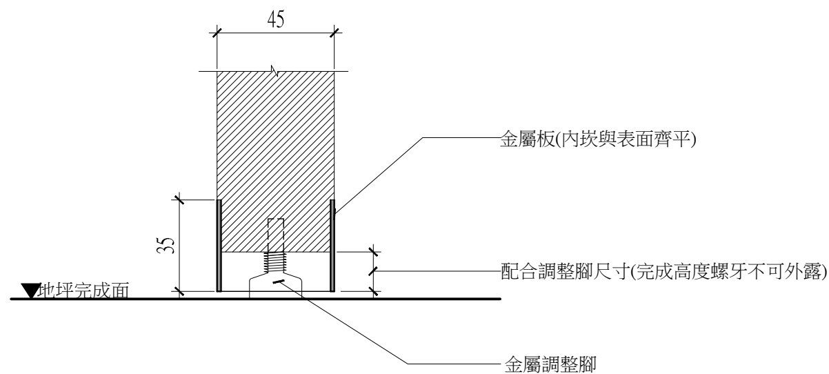
2 大樣圖 1:2
