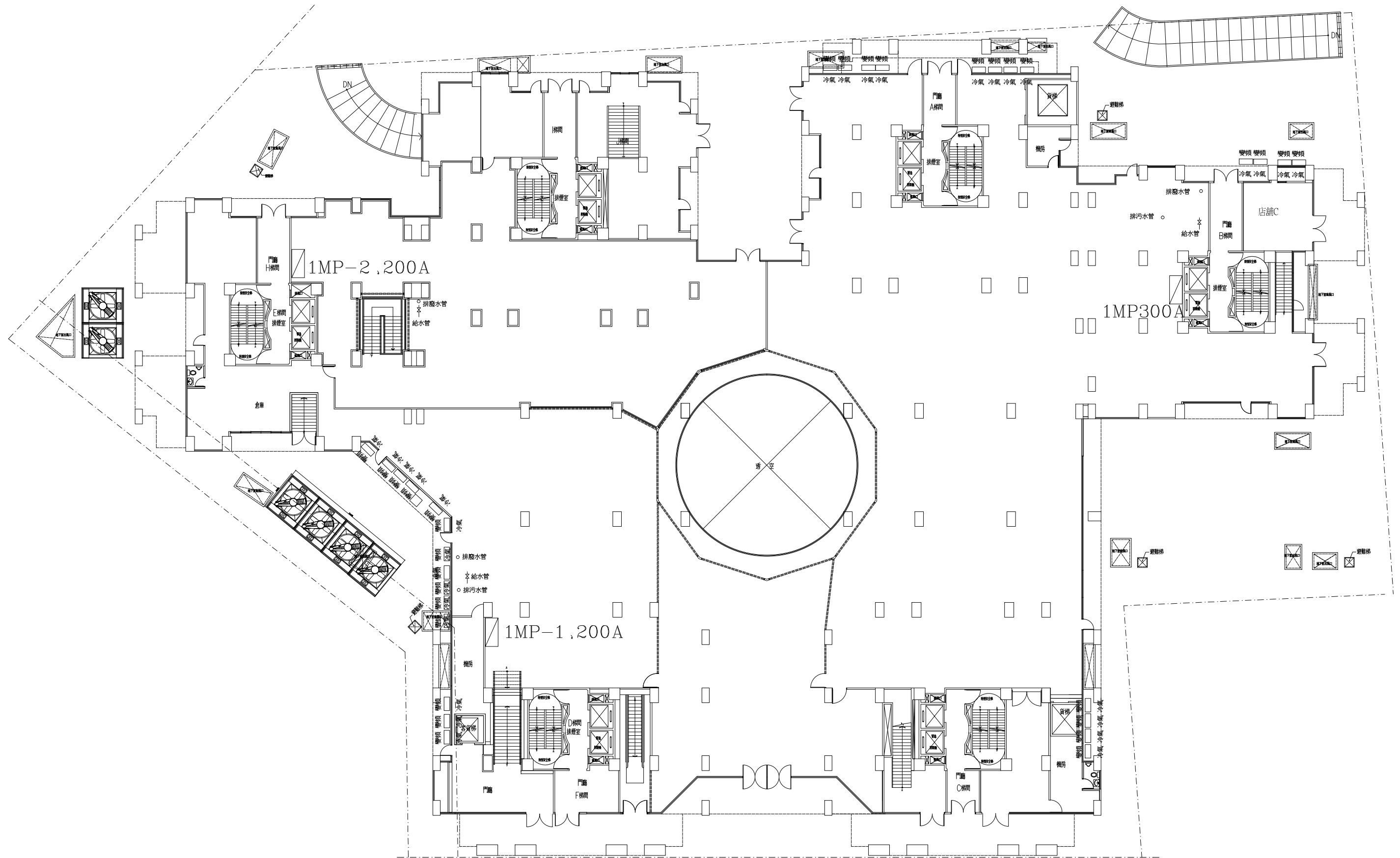
壹層暨室內裝修平面圖
